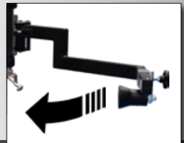
Rullo premi-tallone con regolazione in profondità e ritorno automatico. Adjustable bead pressing roller with automatic return system.
